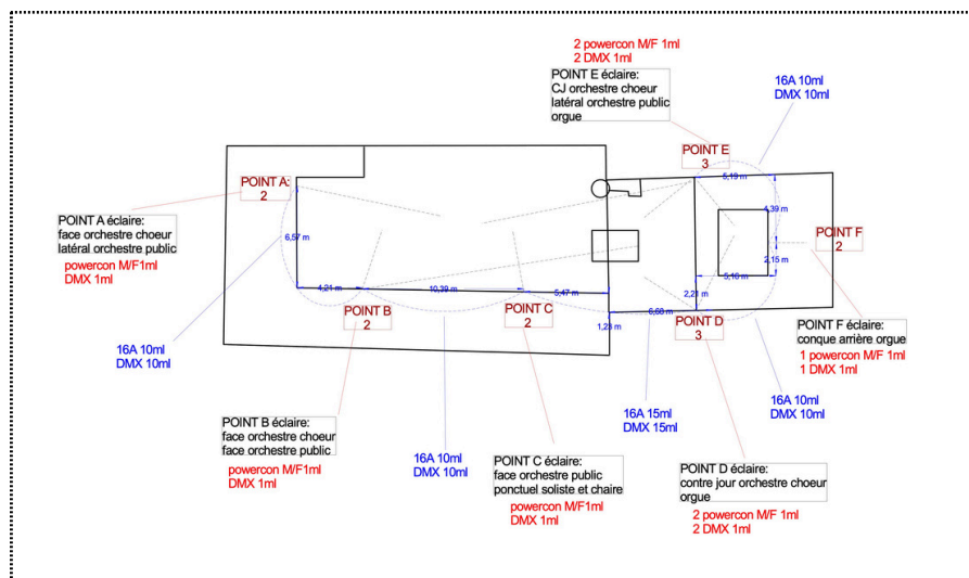
plan d'implantation de l'éclairage
